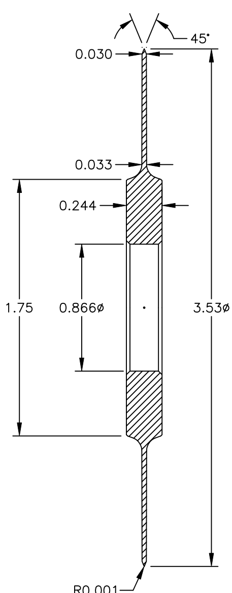
SECTION A-A
