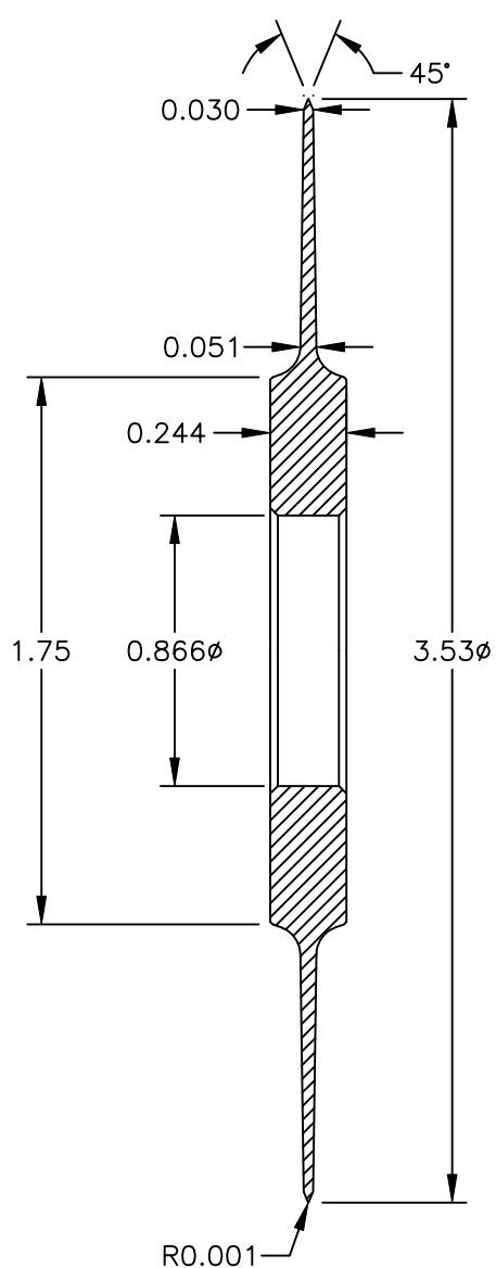
SECTION A-A
