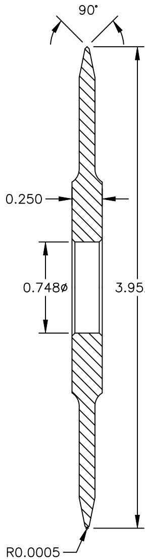
SECTION A-A
